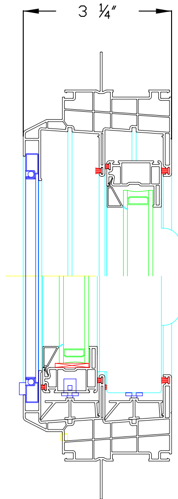
Section A-A
